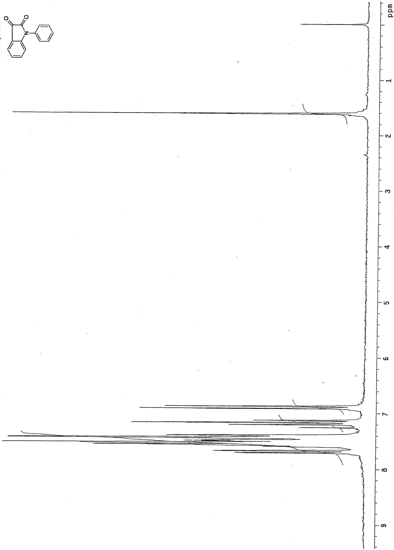
N-Phenylisatin
