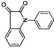
N-Phenylisatin
